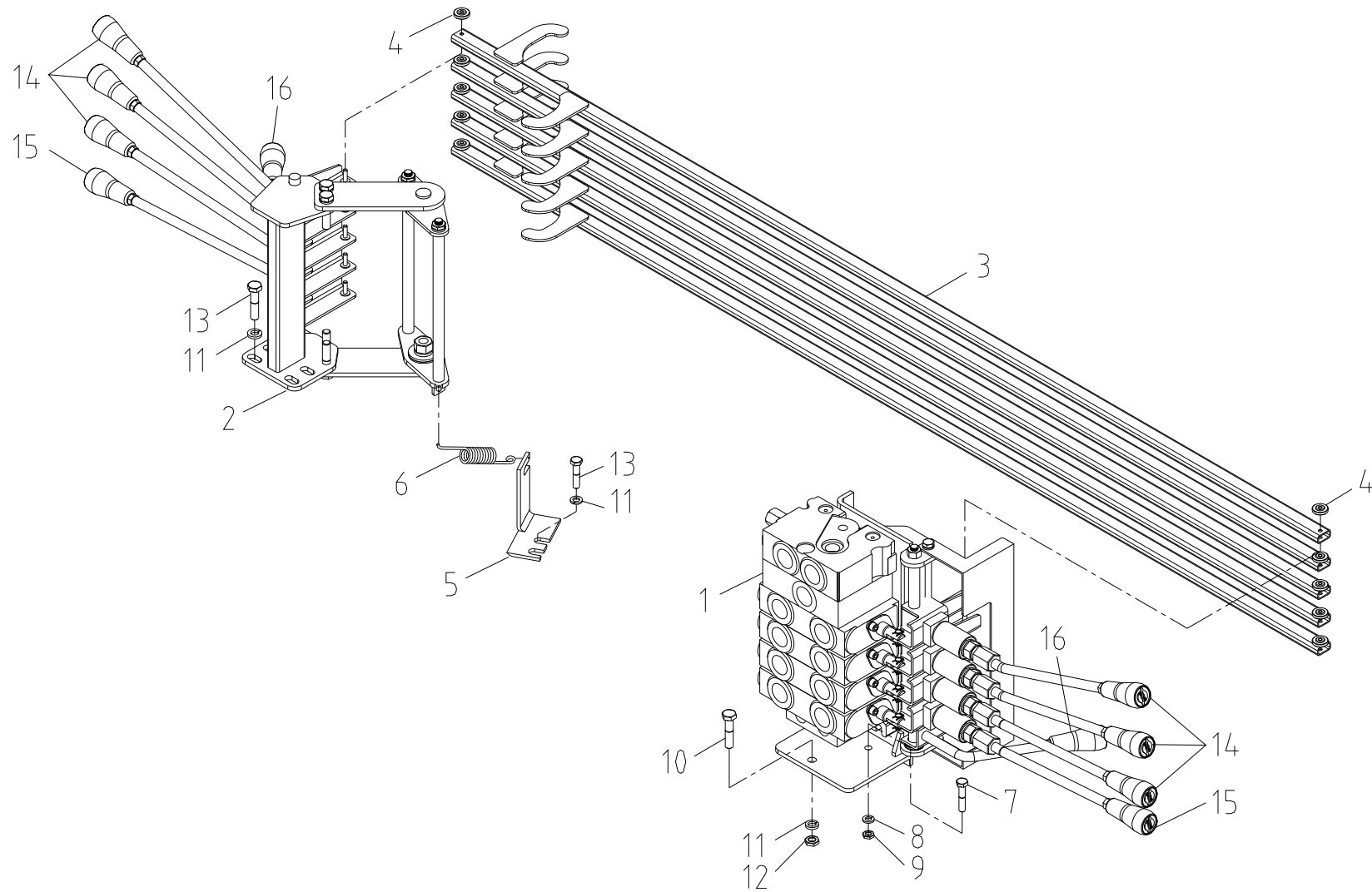
오퍼레이션 메인 조립체 Fig. 3-3 SCS736 OPERATION MAIN ASS'Y
