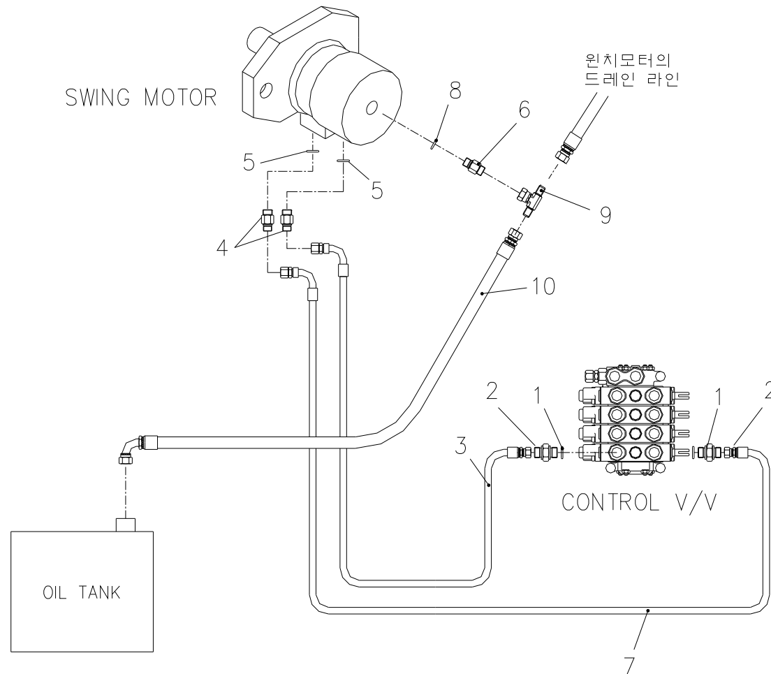
스윙 배관 Fig. 5-5 SCS736 SWING PIPING
