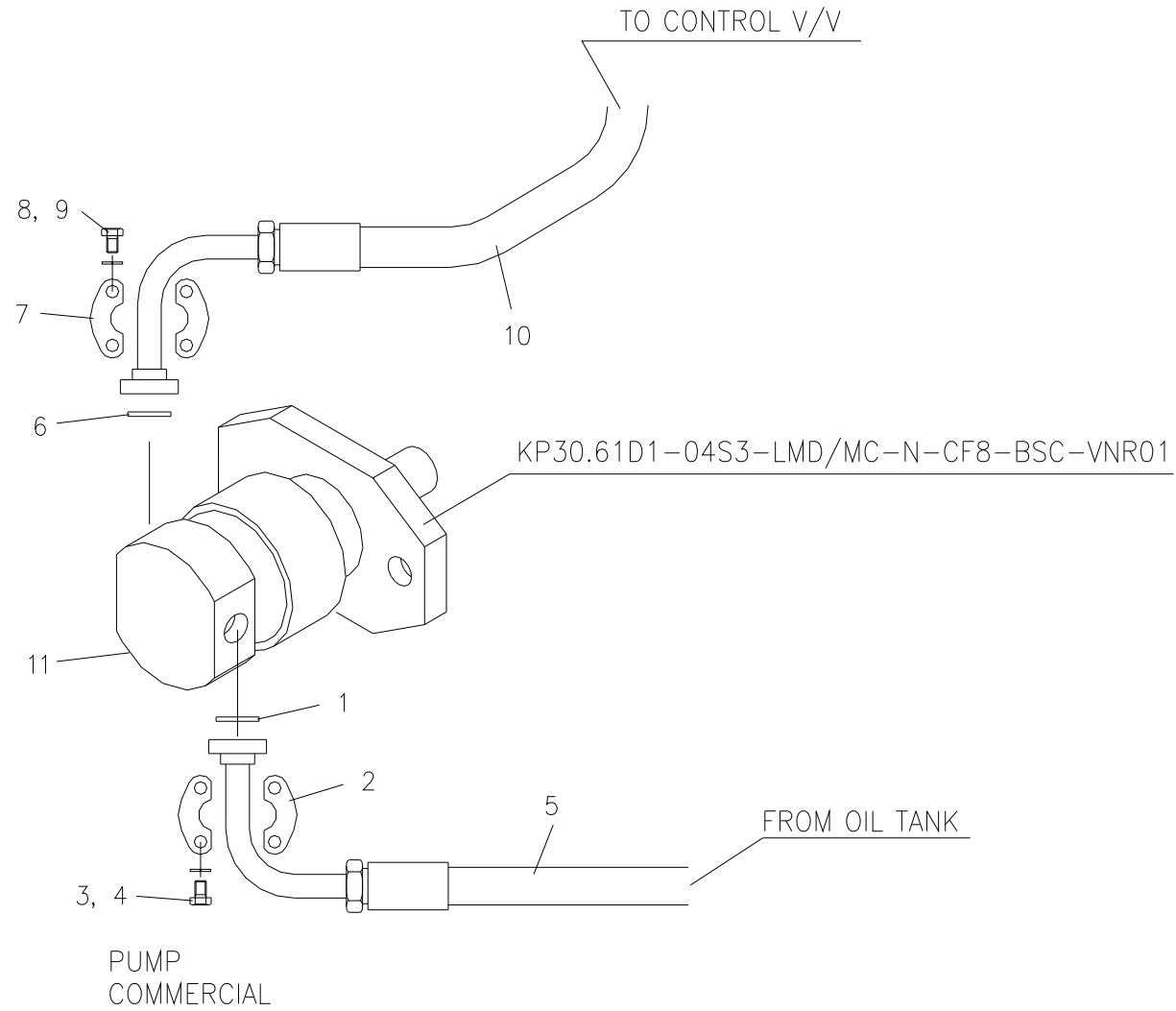
장착 배관 파트 Fig. 8 SCS736 M/T PIPING PART
