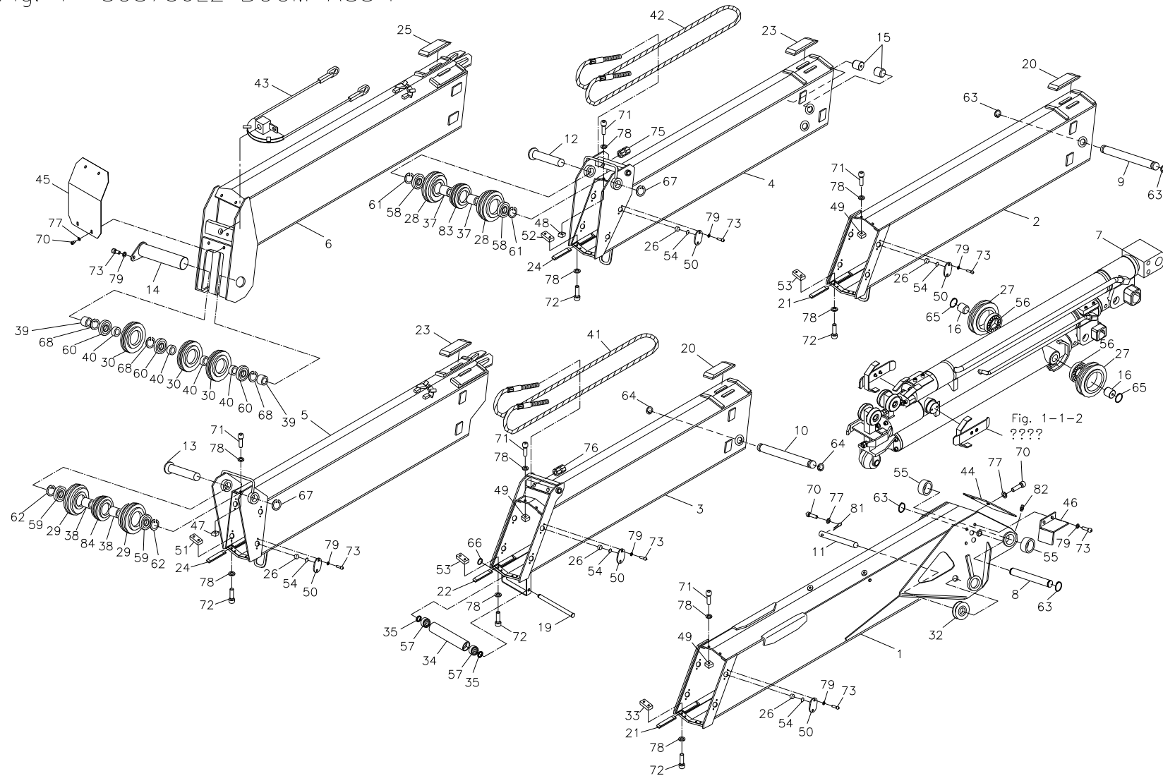
붐 조립체 Fig. 1 SCS736L2 BOOM ASS'Y
