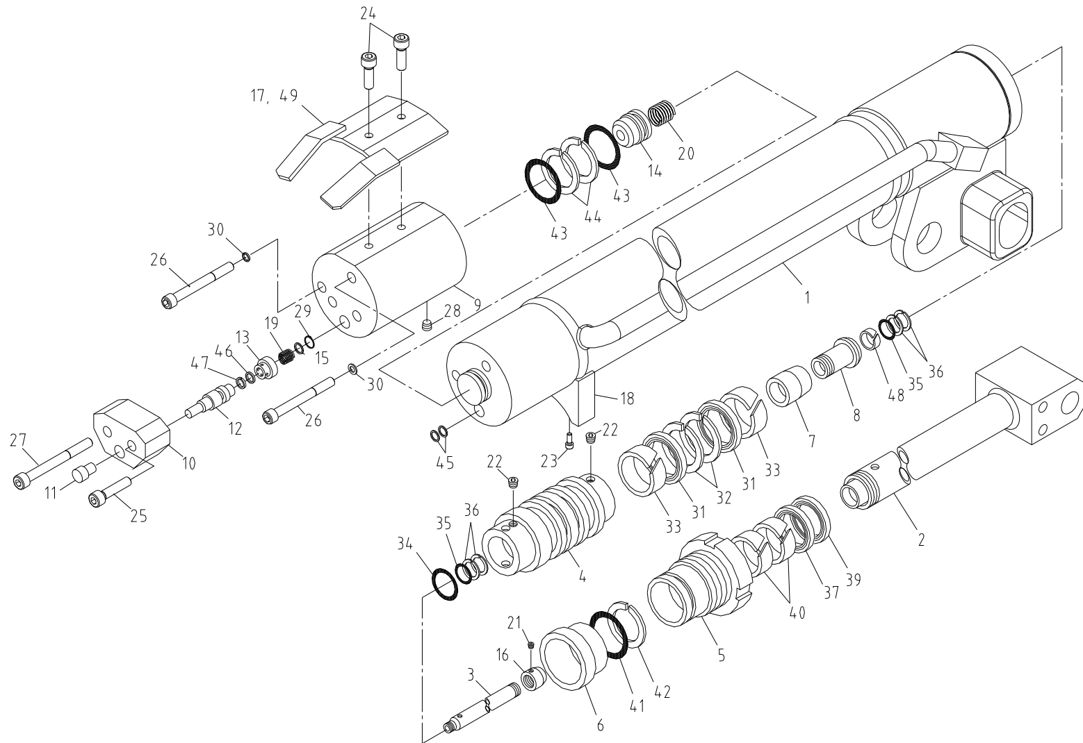
텔레스코픽 실린더(1단) 조립체 (표준형) Fig. 1-1-1 SCS736L2 TELESCOPIC CYL'(1st) ASS'Y (STD)
