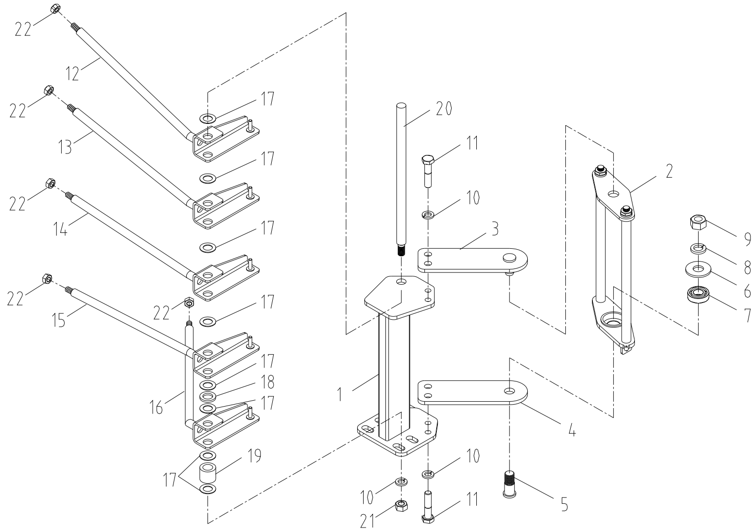
레버 스탠드 세트 Fig. 3-3-2 SCS736 LEVER STAND SET
