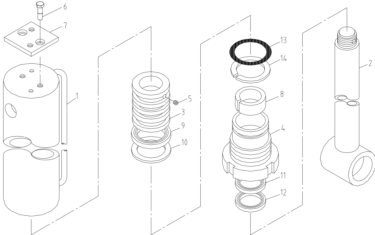
잭 실린더 조립체 Fig. 4-1 SCS736 JACK CYL' ASS'Y
