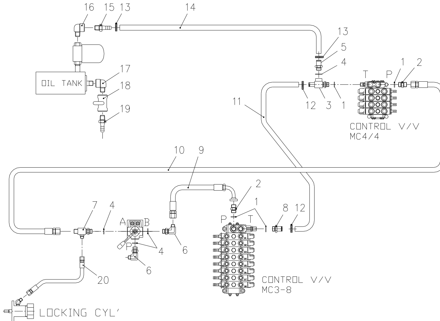
디스트리뷰터 배관 Fig. 5-1 SCS736 DISTRIBUTOR PIPING
