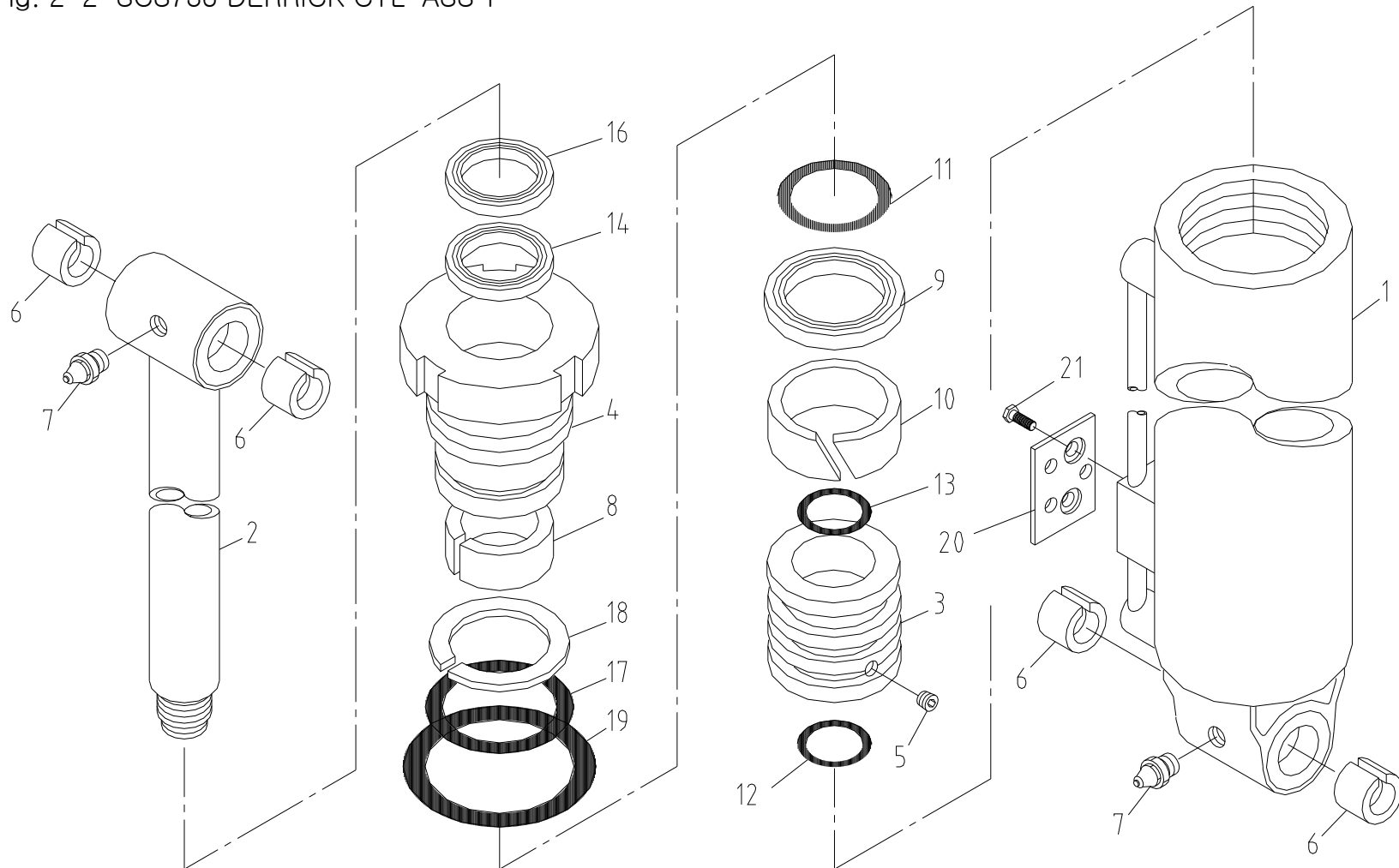
데릭 실린더 조립체 Fig. 2-2 SCS736 DERRICK CYL' ASS'Y
