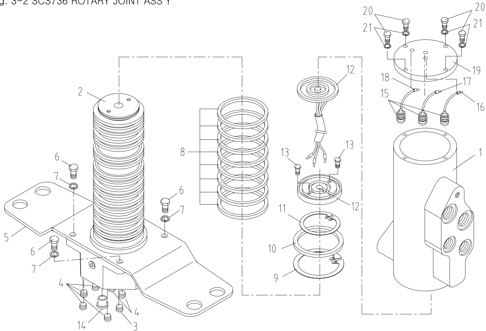
로타리 조인트 조립체 Fig. 3-2 SCS736 ROTARY JOINT ASS'Y
