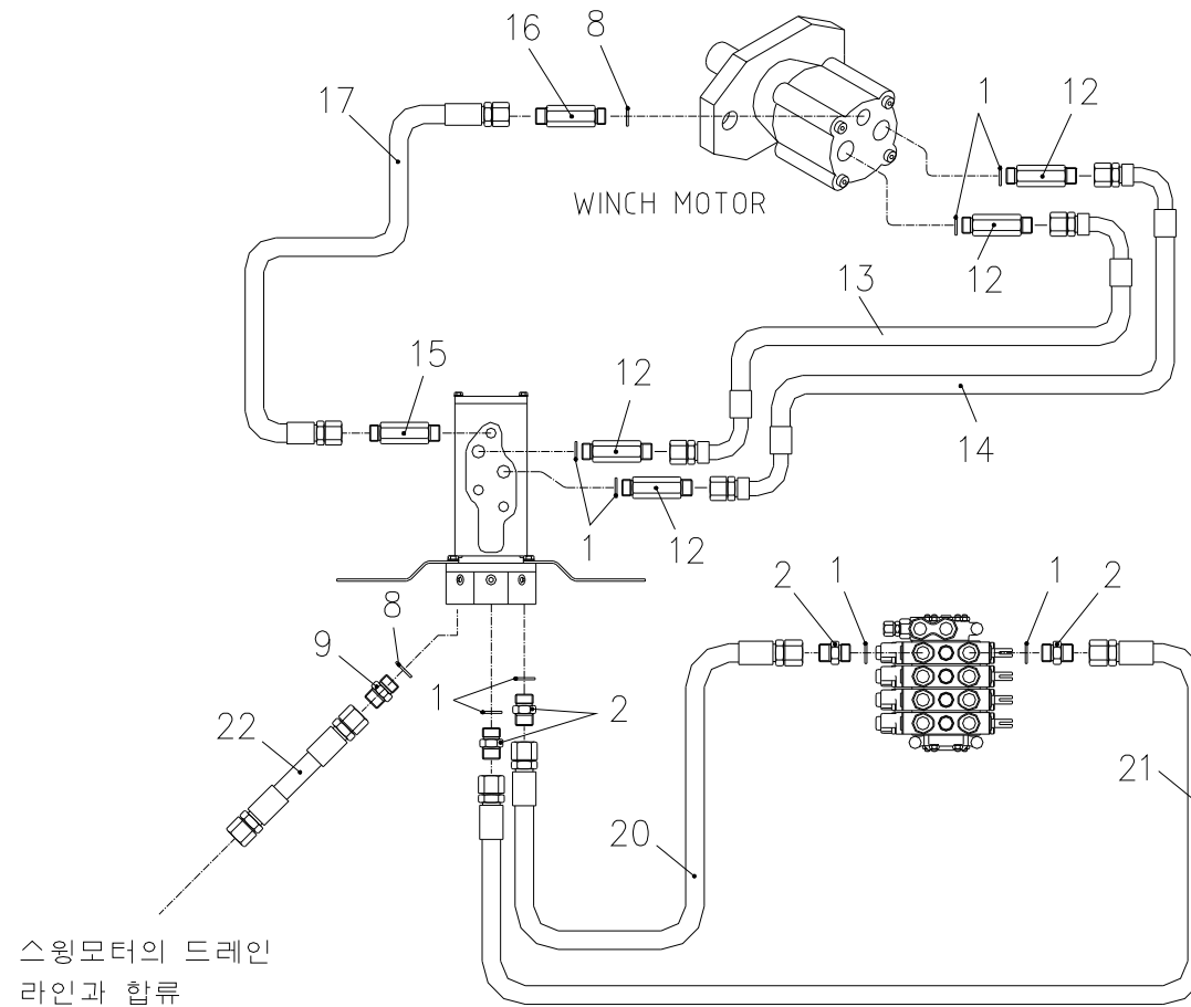
원치 배관 Fig. 5-3 SCS736 WINCH PIPING
