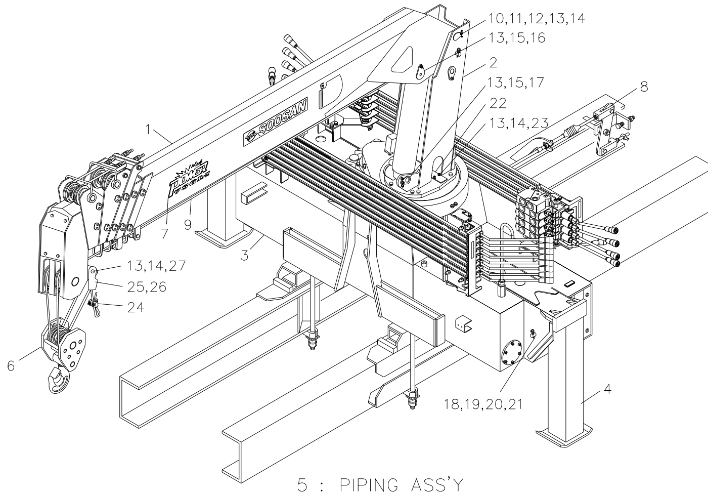
크레인 조립체 Fig. 0 SCS736L2 CRANE ASS'Y
