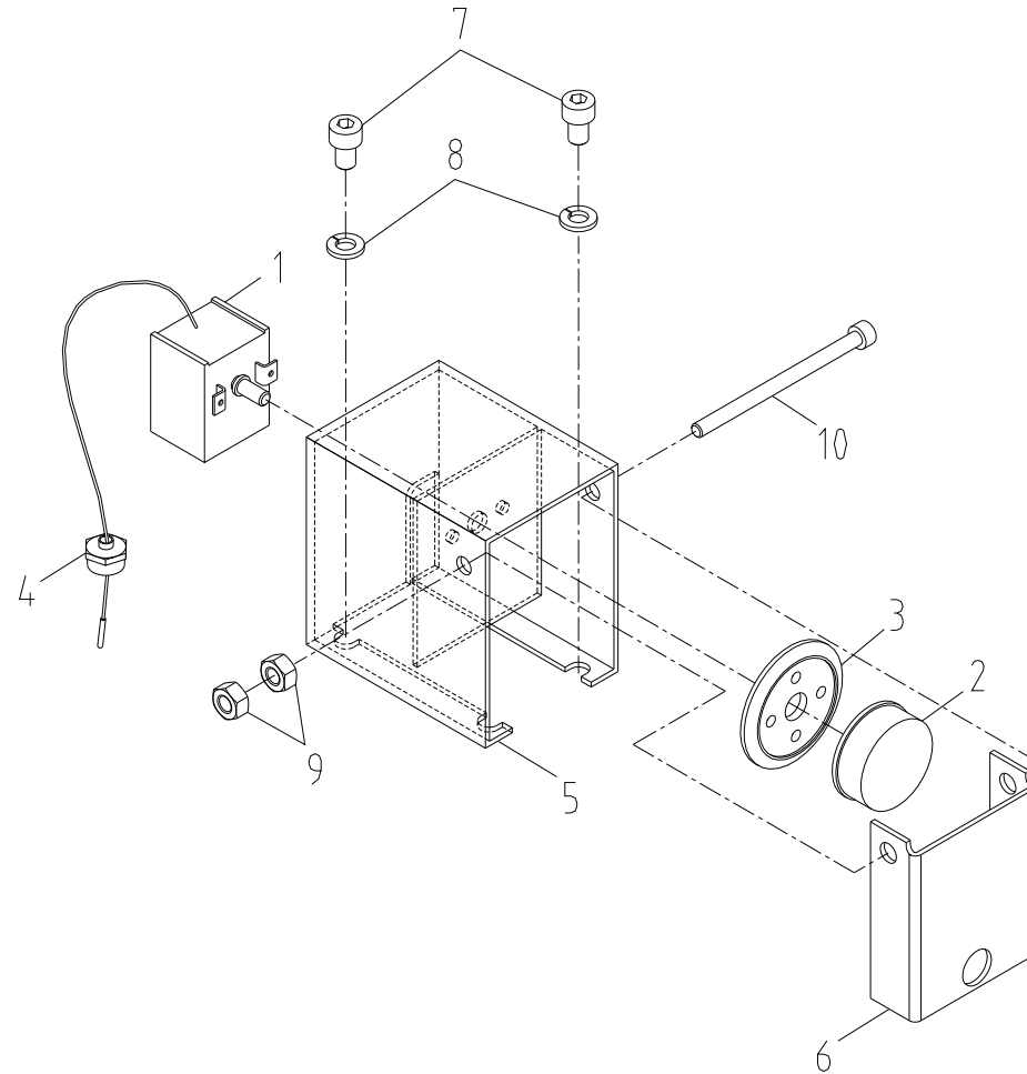
온도 스위치 조립체 Fig. 3-6 SCS736 TEMPERATURE SWITCH ASS'Y
