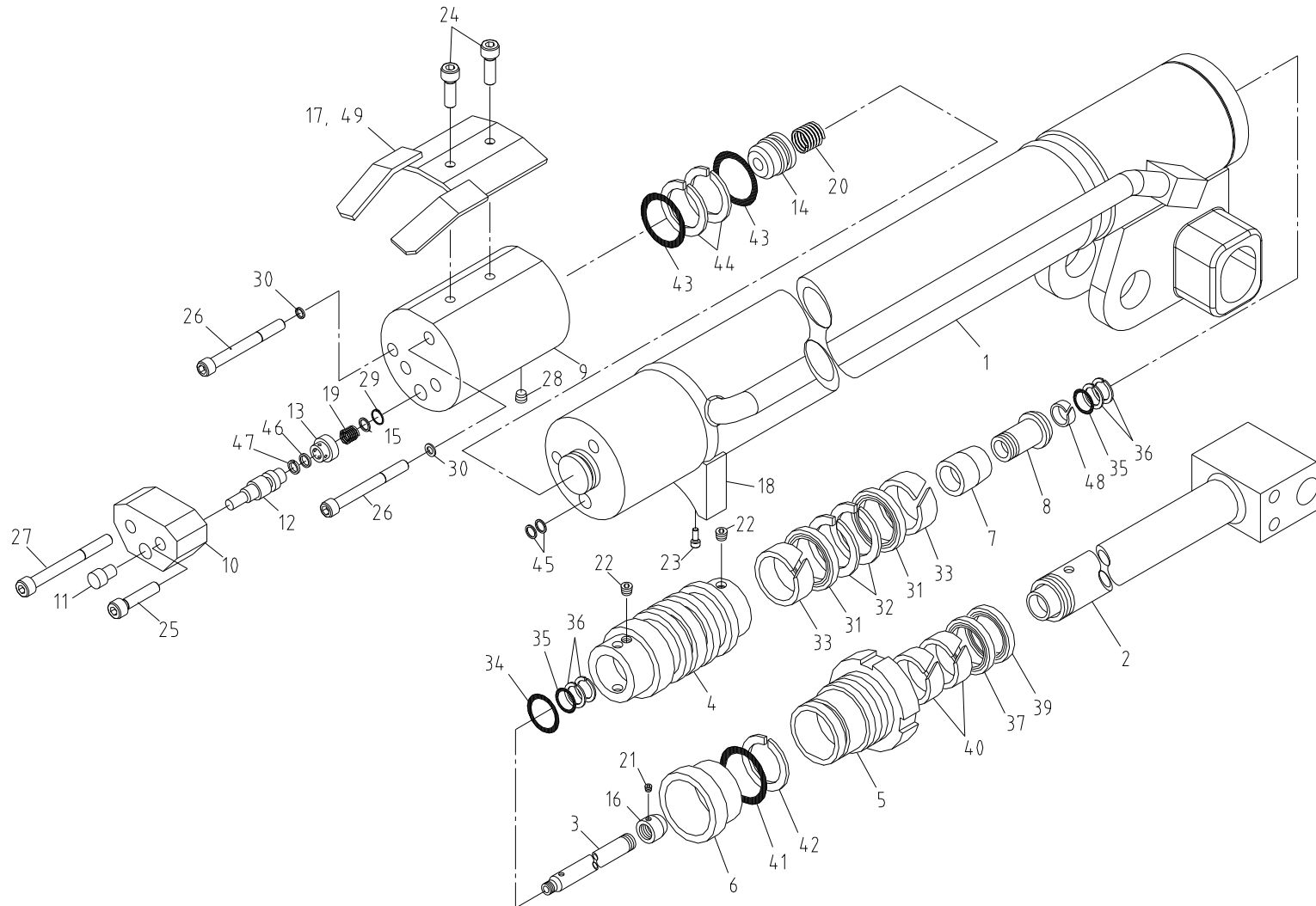
텔레스코픽 실린더(1단) 조립체 (표준형) Fig. 1-1-1 SCS736 TELESCOPIC CYL'(1st) ASS'Y (STD)
