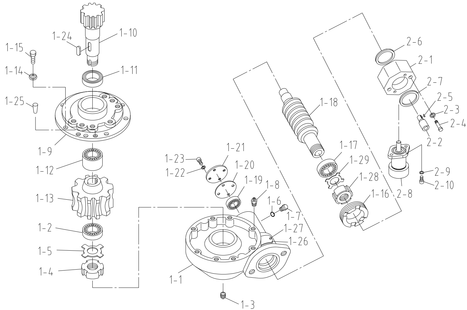
스윙 감속기 셋트 Fig. 3-1 SCS736 SWING R/G SET
