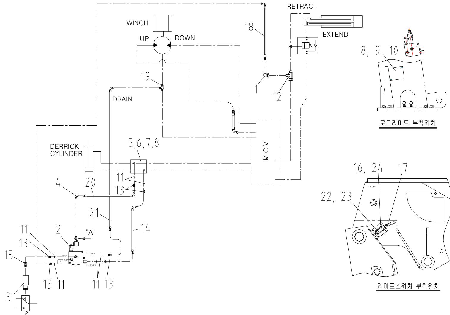
과하중 방지 배관 조립체 Fig. 10 SCS736 OVERWINDING ALARM PIPING ASS'Y
