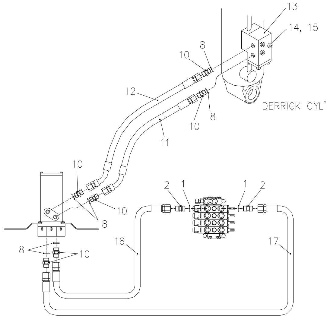
데릭 배관 Fig. 5-2 SCS736 DERRICK PIPING
