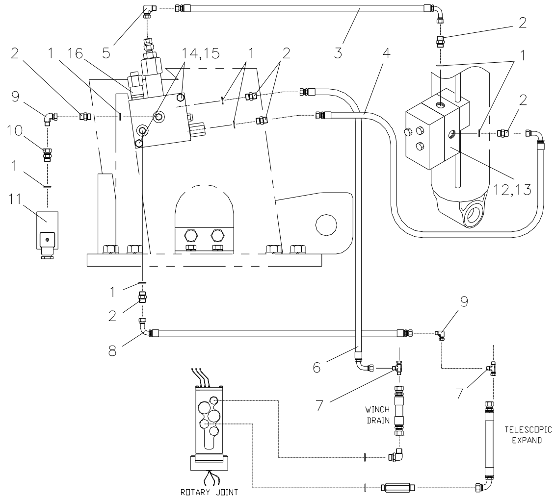
로드 리미트 배관 Fig. 5-10 SCS736 LOAD LIMMIT PIPING
