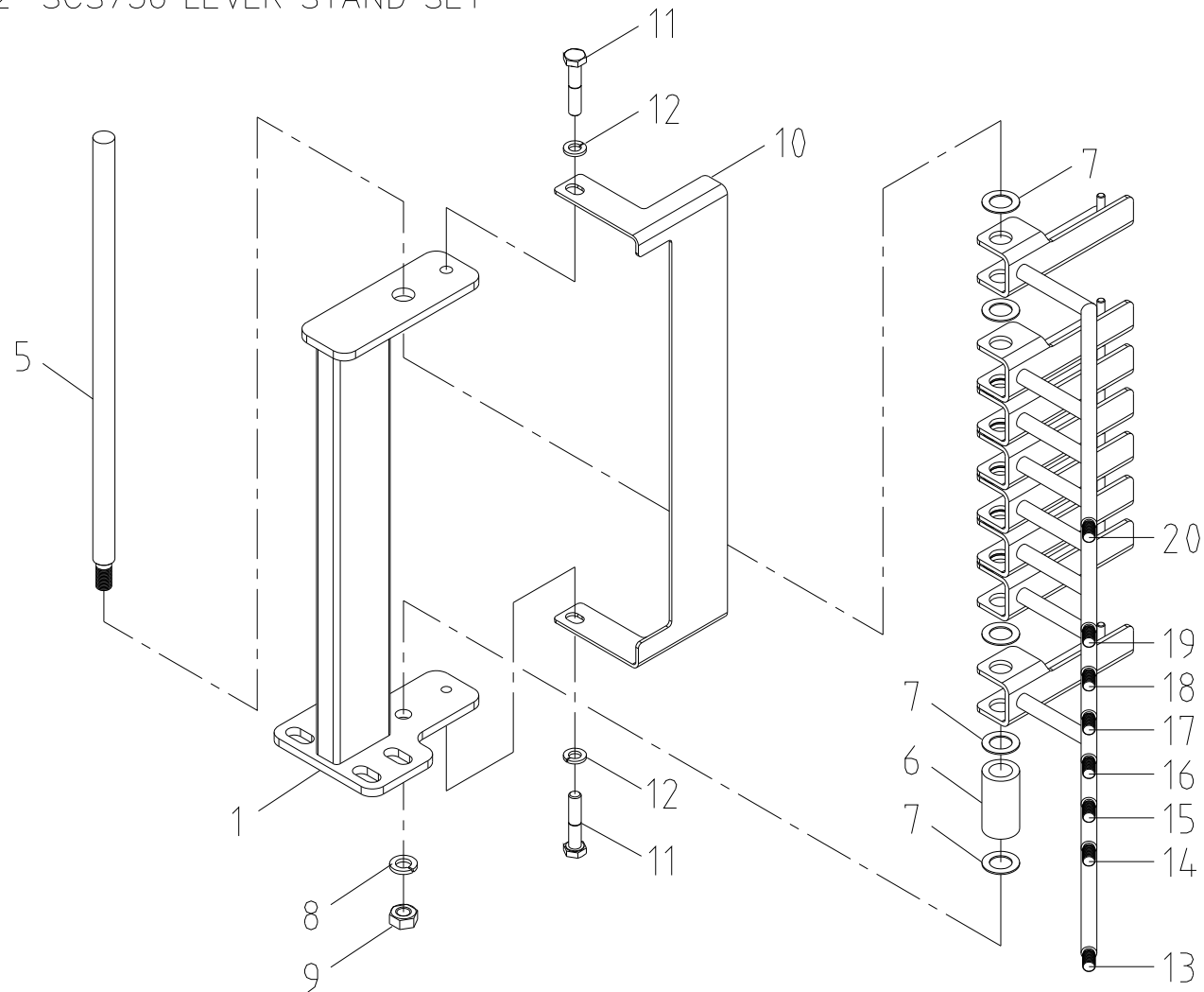
레버 스텐드 셋 Fig. 3-4-2 SCS736 LEVER STAND SET
